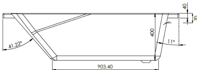
SECTION A-A SCALE 1 : 9
